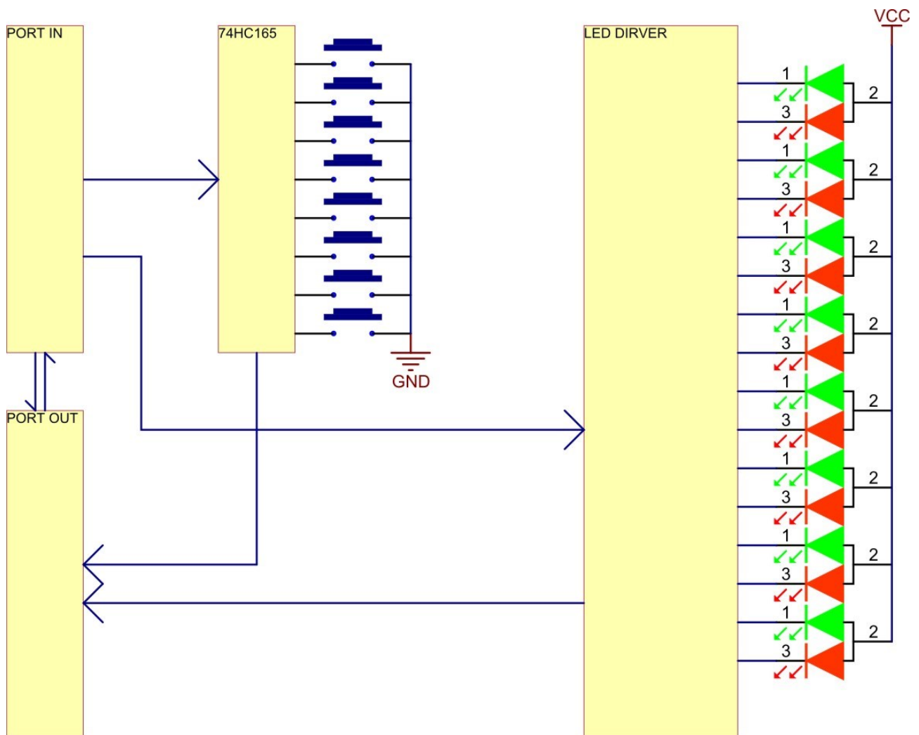
Рис. 4.1. Блок-схема блока расширения микрофонных консолей LPA-EVA-EM
